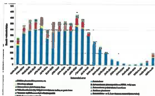
Figura 3.7. Distribuția volumelor de trafic, Post 13 – DN 2G, 24 ore.
